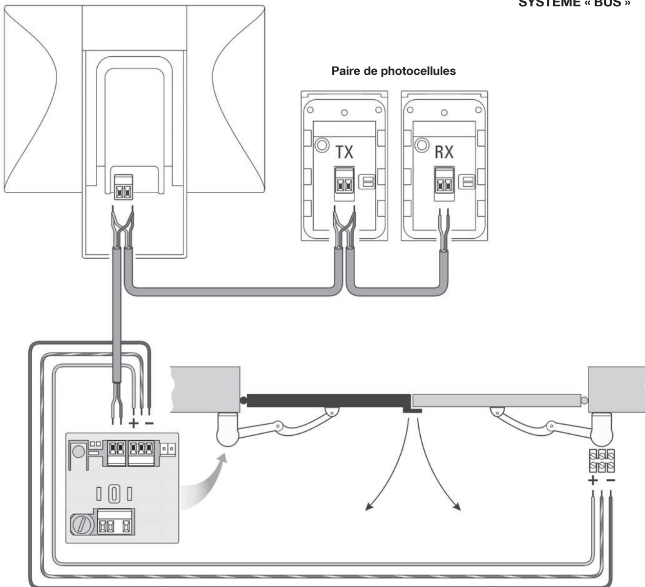
SCHÉMA DE CONNEXION DES DISPOSITIFS AVEC SYSTÈME « BUS »
