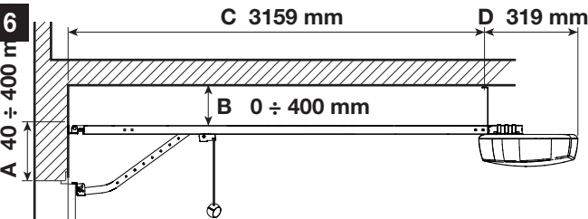
PORTE SECTIONNELLE
