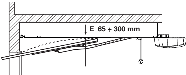
PORTE BASCULANTE DÉBORDANTE PORTE BASCULANTE NON DÉBORDANTE
