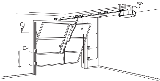
PORTE BASCULANTE NON DÉBORDANTE
